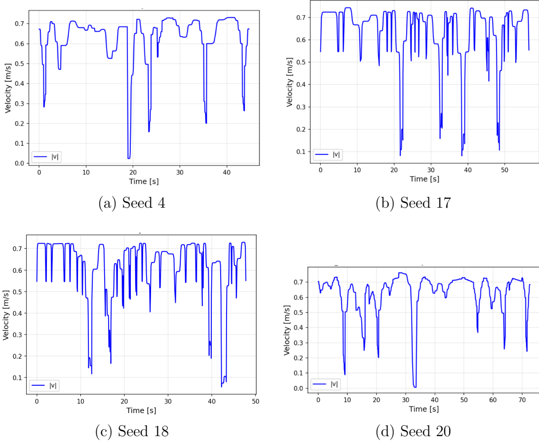
Hình 5.4: Hồ sơ vận tốc của các nghiệm GCS-DMS trong mê cung. Các pha giảm tốc xuất hiện tại những đoạn cua hẹp hoặc chuyển tiếp nhiều vùng, phản ánh tác động trực tiếp của ràng buộc động lực học phi tuyến.
