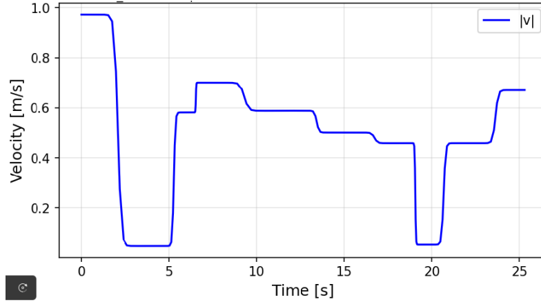
Hình 5.2: Hồ sơ vận tốc của nghiệm GCS-DMS trên môi trường 2D đơn giản. Vận tốc giảm tại các đoạn cua và tăng trở lại ở các đoạn có hình học thuận lợi hơn.
